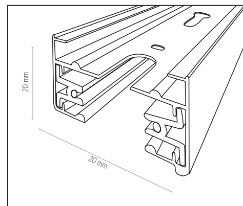
PRZEKRÓJ LISTWY PROWADZĄCEJ
